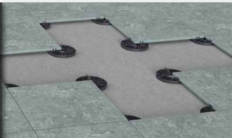
Otworki na motylki dystansowe w podstawkach 8, 10, 15, 16 mm
